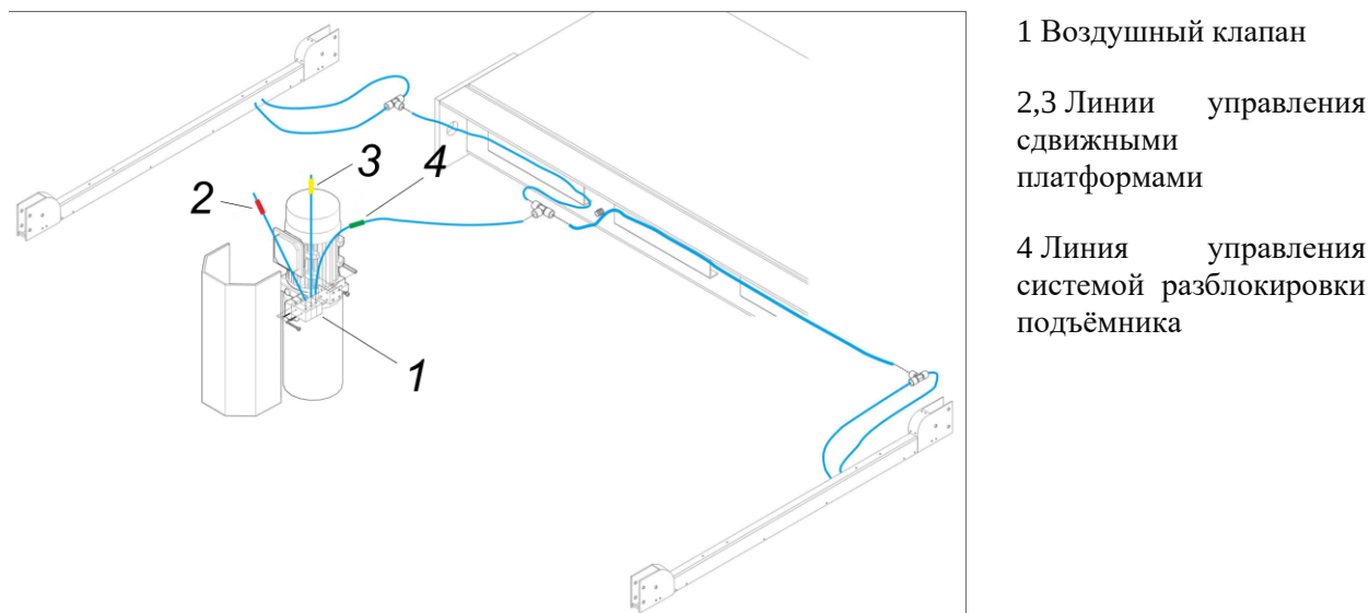
Рисунок 3.13 – Схема подключения пневматической системы разблокирования подъёмника
