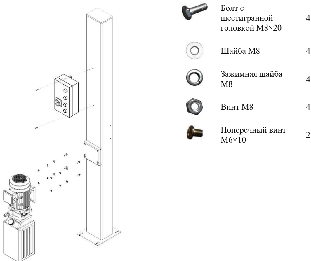
Рисунок 3.11 – Схема установки гидростанции и блока управления
