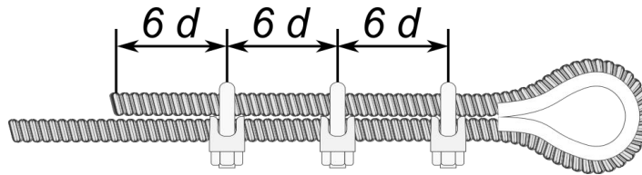
Рисунок 3.10 – Крепление троса с помощью и-образных зажимов
