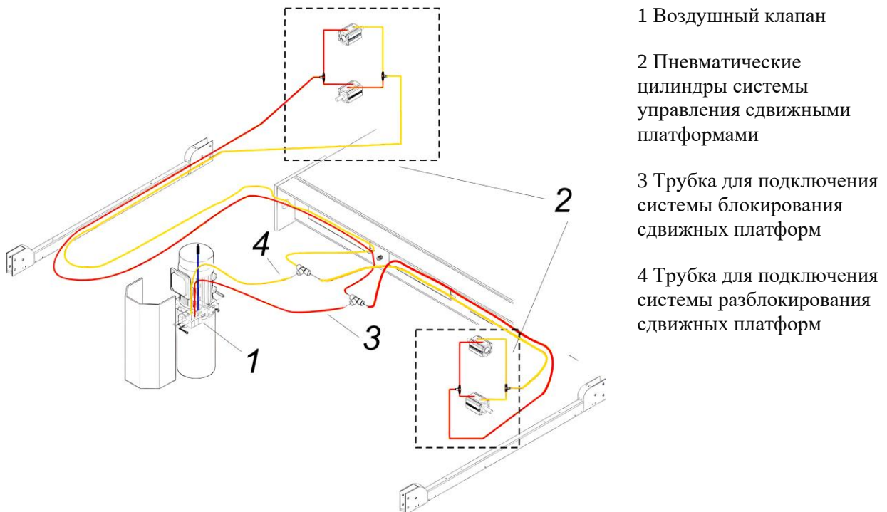
Рисунок 3.14 – Схема подключения пневматической системы управления сдвижными платформами
