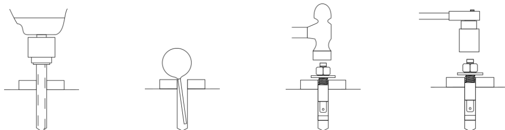
Рисунок 3.22 – Установка анкерных болтов
