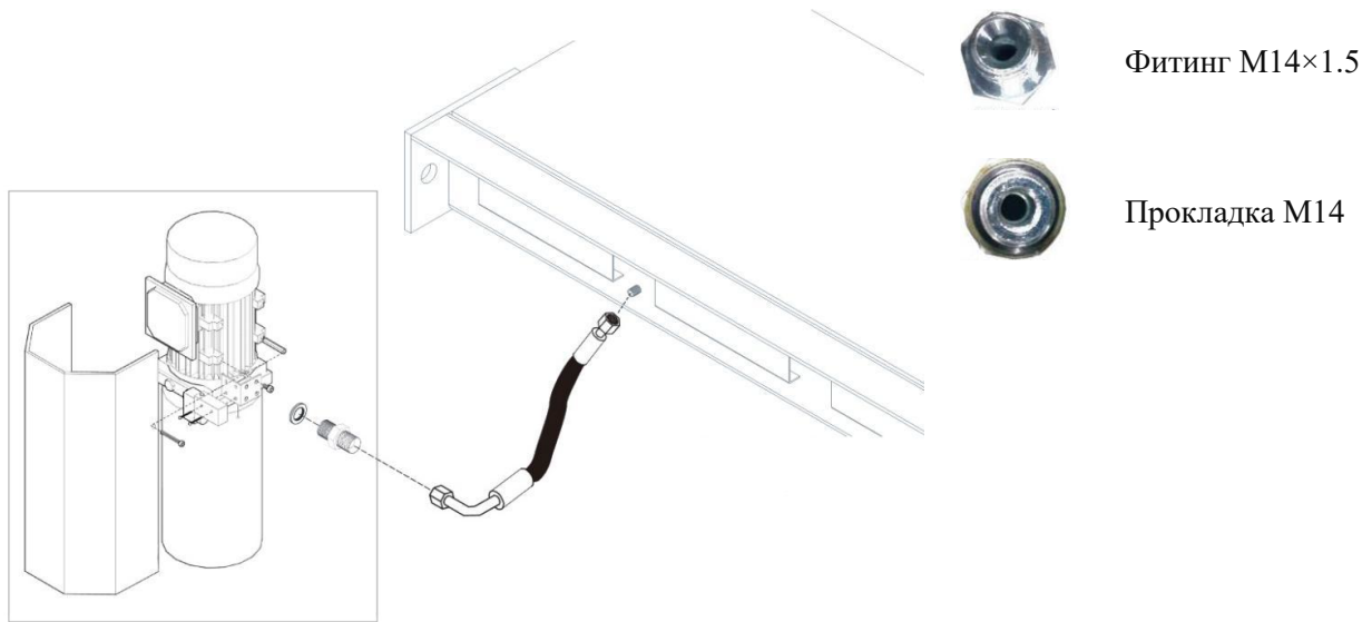
Рисунок 3.12 – Схема подключения гидростанции
