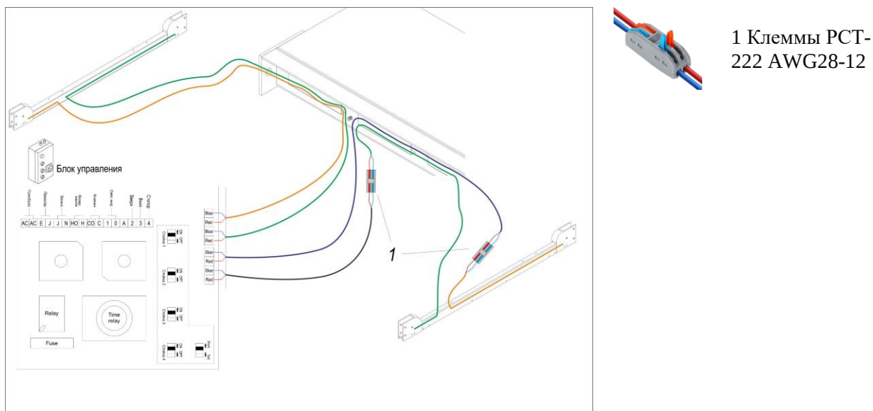
Рисунок 3.19 – Схема подключения датчиков положения
