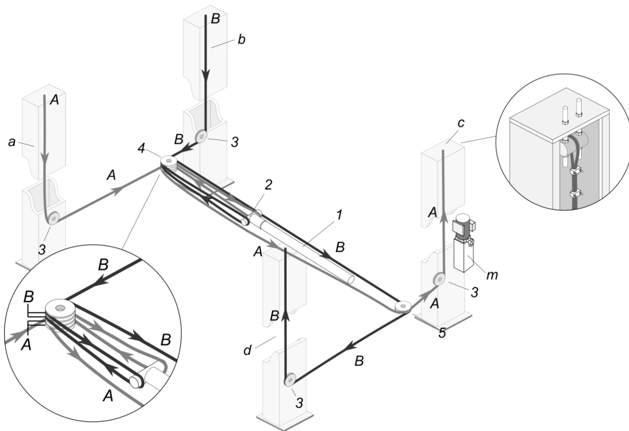
Рисунок 3.9 – Устройство подъёмного механизма
