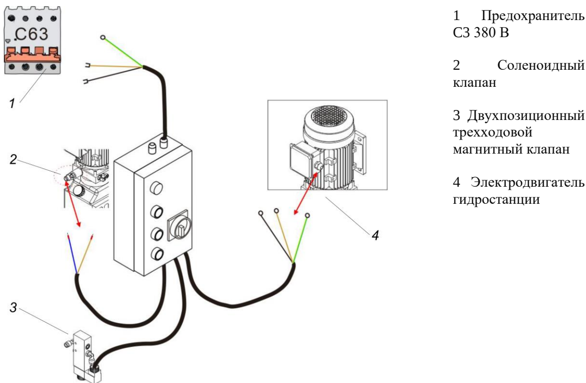
Рисунок 3.15 – Общая схема подключения блока управления
