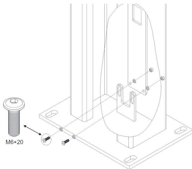
Рисунок 3.6 – Закрепление стопорных реек снизу
