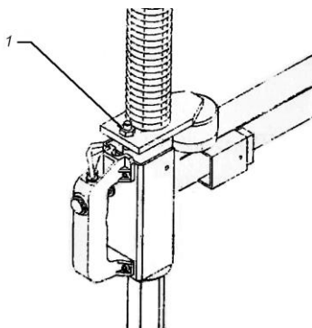
Рисунок 6.4 – Регулировка болта
